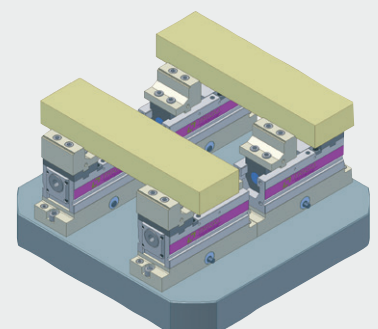
4 x Schnellspannwechselblock Größe 1 (Sonder) und 4x SCS 80-200 auf Palette 540 x 540 mm
