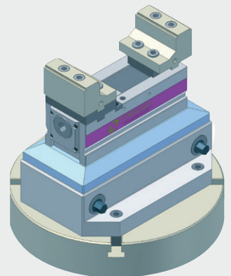
Schnellspannwechselblock Größe 2 mit SCS 80-200 und Adapterplatte
