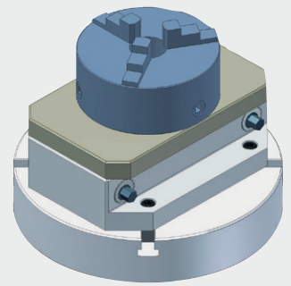
Schnellspannwechselblock Größe 2 mit Dreibackenfutter und Adapterplatte
