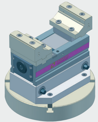
Schnellspannwechselblock Größe 2 mit SCS 120-250 auf Rundtisch
