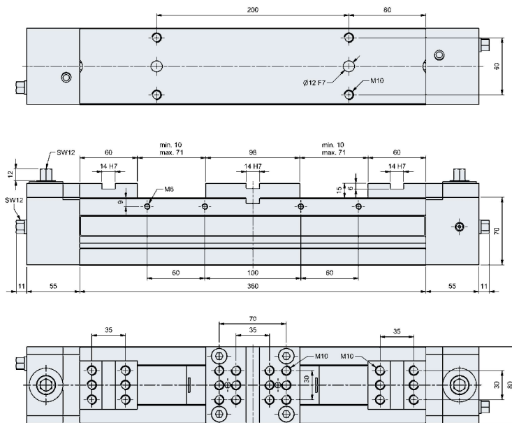
Spannbereich mit Wende- und Mittenbacke sowie Stufenwende- und Stufenmittelbacke
