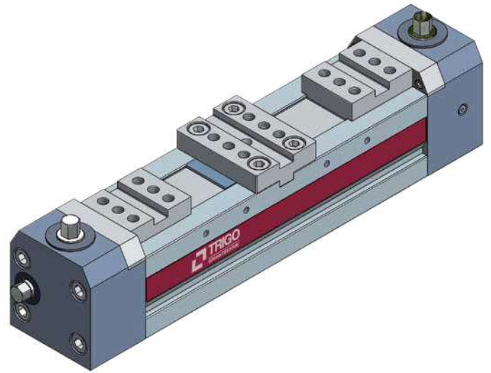
Spannbereich mit Wende- und Mittenbacke sowie Stufenwende- und Stufenmittelbacke
